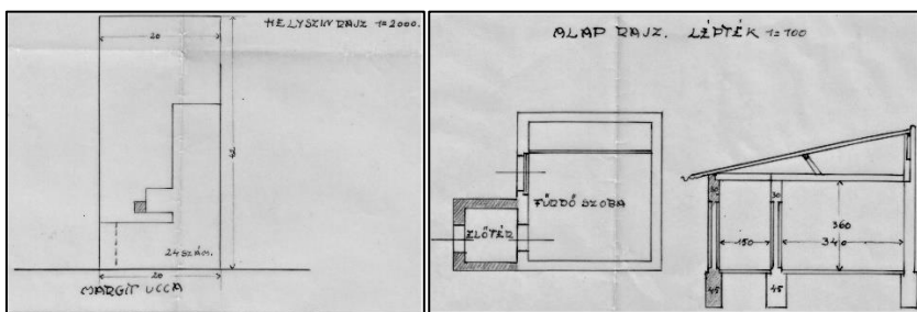
A rituális fürdő előszobája építésének tervei
